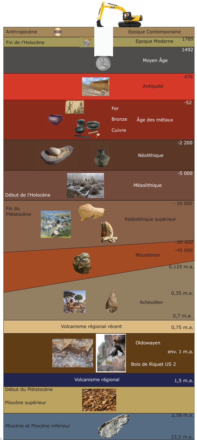
Stratigraphie simplifiée
